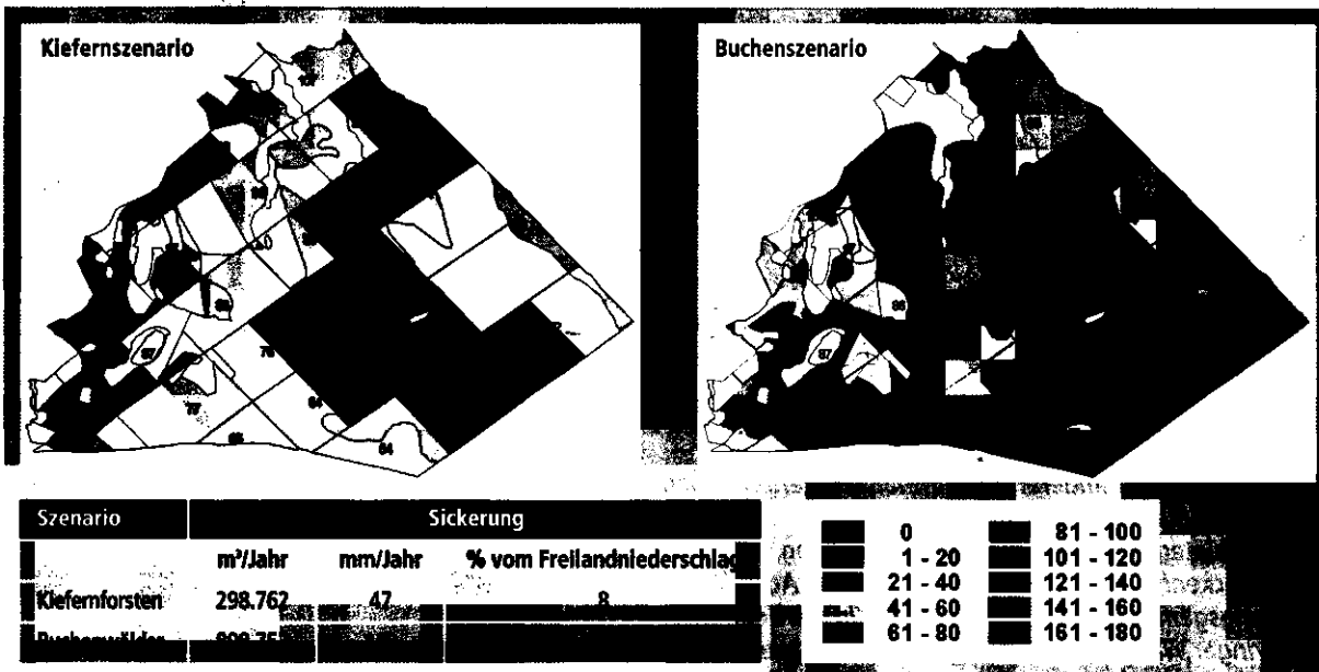
Abb. 4: Tiefensickerung bei unterschiedlicher Waldbestockung am Beispiel eines Forstreviers auf der Talsandterrasse des Choriner Endmoränenbogens (642 ha; 620 mm Jahresniederschlag)
